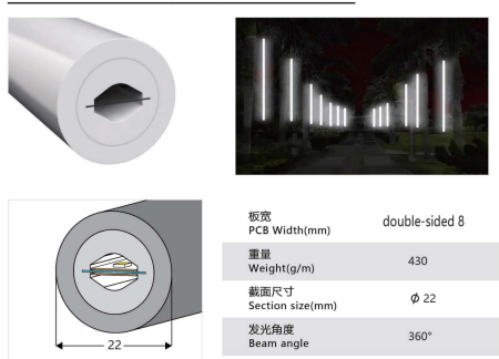
Side View \phi 22 (mm)360°B 防断款
