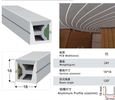
Side View 16*16(mm) 防断款
