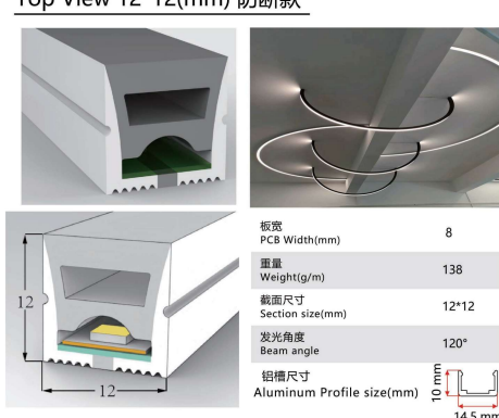
Top View 12*12(mm) 防断款
